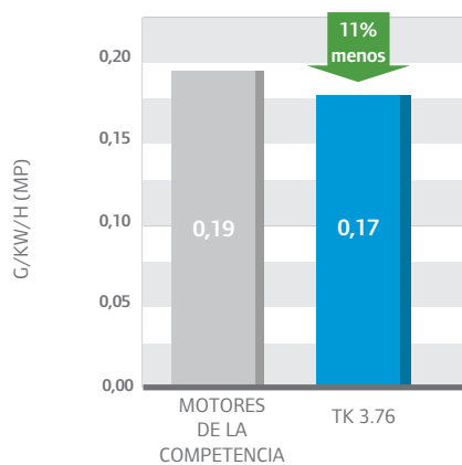
EMISIONES (MATERIA PARTICULADA): LOS MOTORES DE LA COMPETENCIA FRENTE A LOS DE LA SERIE UT
